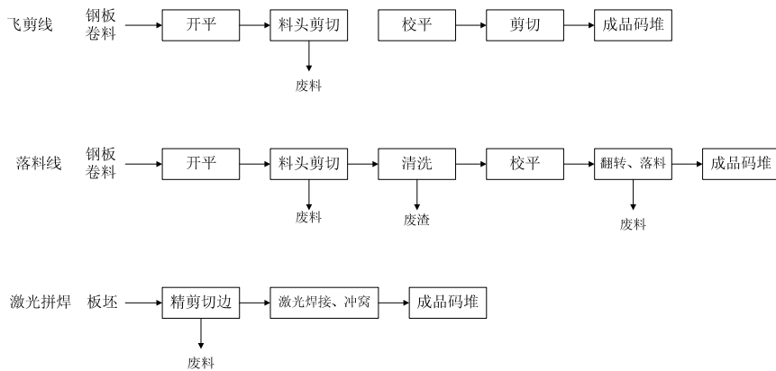
图 1 生产工艺及污染流程图
